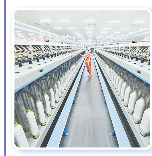
↑5月30日，焦作市汇百川纺织有限公司工人在纺纱。该公司位于博爱经济技术开发区，总投资1.2亿元的年产9500吨高档精品纱线项目，目前一期已完成，二期正在施工。项目全部建成后，可实现销售收入2.5亿元，利税1500万元。 本报记者 刘金元 摄
