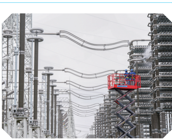
世界最高电压等级换流站完成“体检”。日前,国网安徽电力检修人员对古泉换流站设备进行检修、维护。当日,昌吉-古泉±1100千伏特高压直流输电线路的受端站——安徽宣城古泉换流站完成“体检”。连日来,国网安徽电力的700多名电力检修人员对古泉换流站进行集中检修,有序完成39个作业面共计5200余项工作,为电网的安全稳定运行打下坚实基础。 摘自新华社
