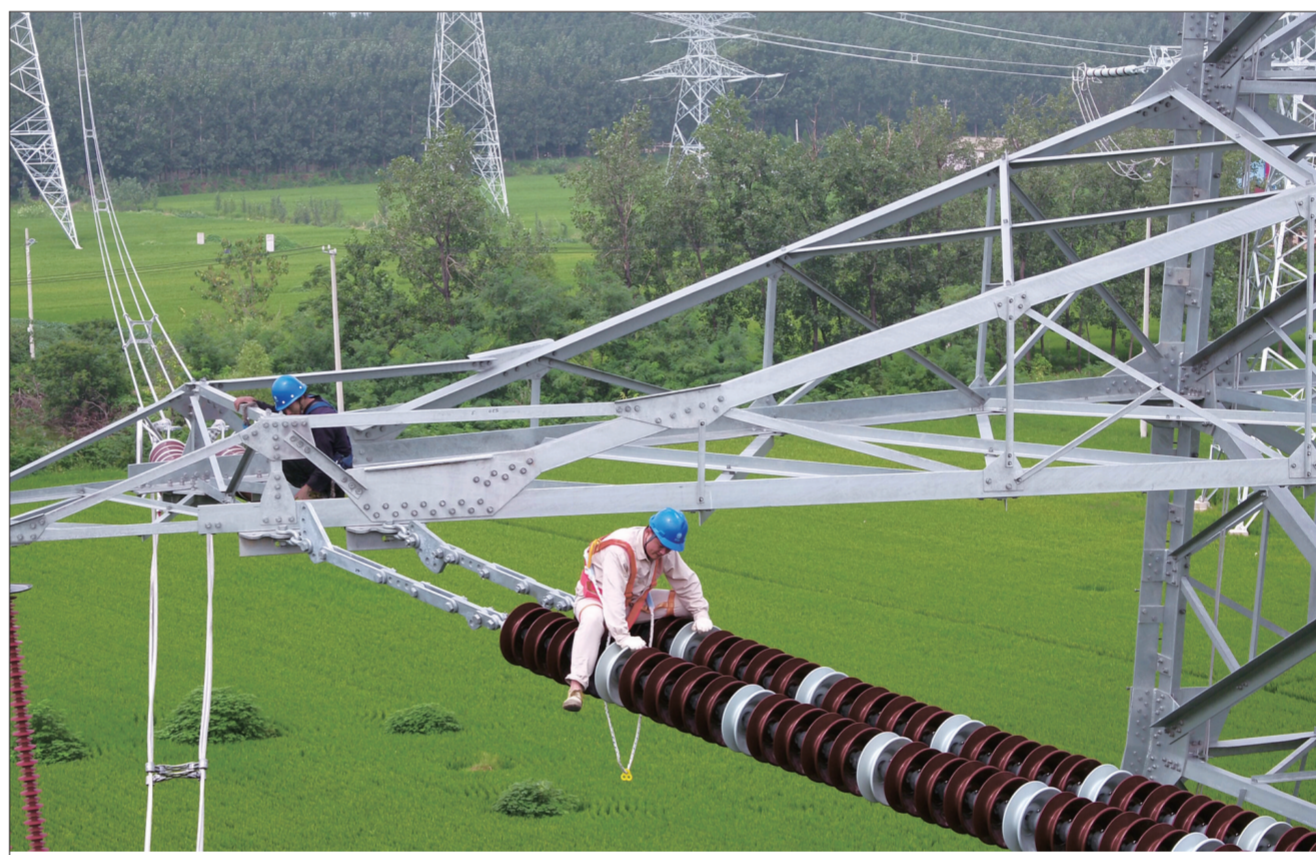
9月7日,国网江苏检修公司员工正在对新建的500千伏伏集/黄堡线路进行投运前的验收。该线路是220千伏黄集变电站升压为500千伏变电站工程的一部分,预计11月建成投运,届时将进一步完善徐州西北部电网结构。 王旭光 褚红雷 摄文
