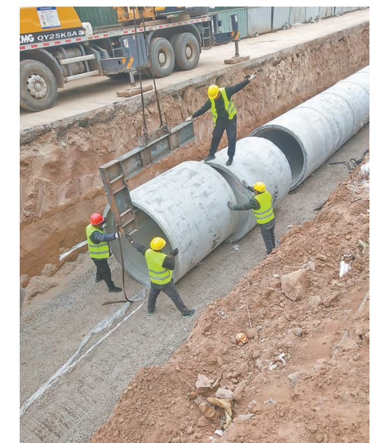
近日，武陟县黄河大道改造工程在进行雨水管网敷设安装工程。该项目总投资8546万元，全长3237米，设计为双向六车道，主要改造内容包括道路、雨污分流、照明、热力、通信等工程。
