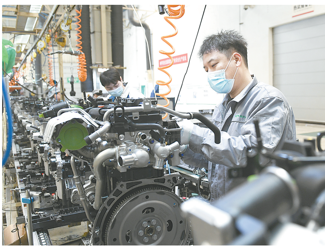
3月30日，瑞庆汽车发动机技术有限公司工人在组装发动机。连日来，该公司在认真落实疫情防控措施的情况下，加快复工复产步伐，各条生产线工人迅速返岗恢复生产，力争实现首季“开门红”。本报记者 刘金元 摄
