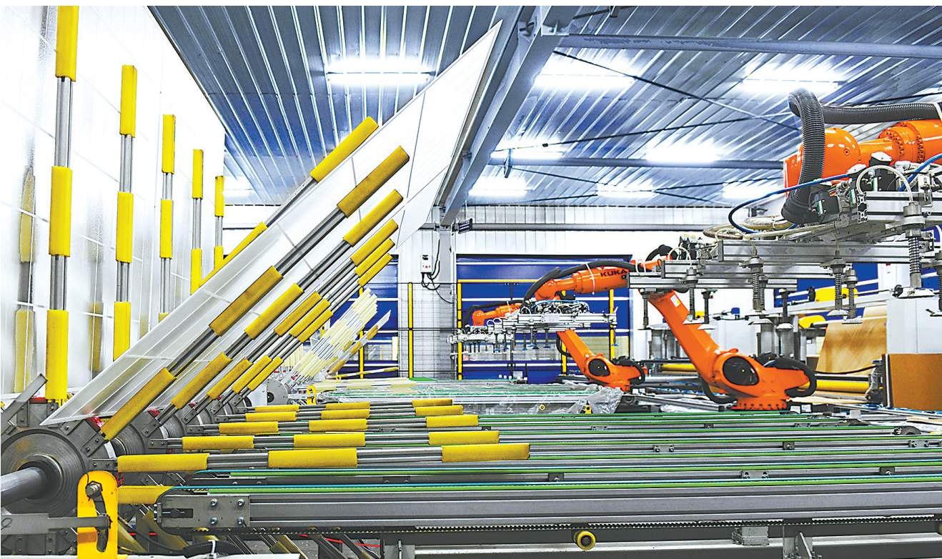
2月18日，位于博爱经济技术开发区的焦作安彩新材料有限公司自动化生产线机器人在生产镀膜强化光伏玻璃。该公司致力于建设既能又环保型低排放企业，加大设备改造升级力度，改造后的光伏玻璃在市场上供不应求，深受客户欢迎，设备从原来年排放氮氧化合物880吨，也降低到76吨以下。
