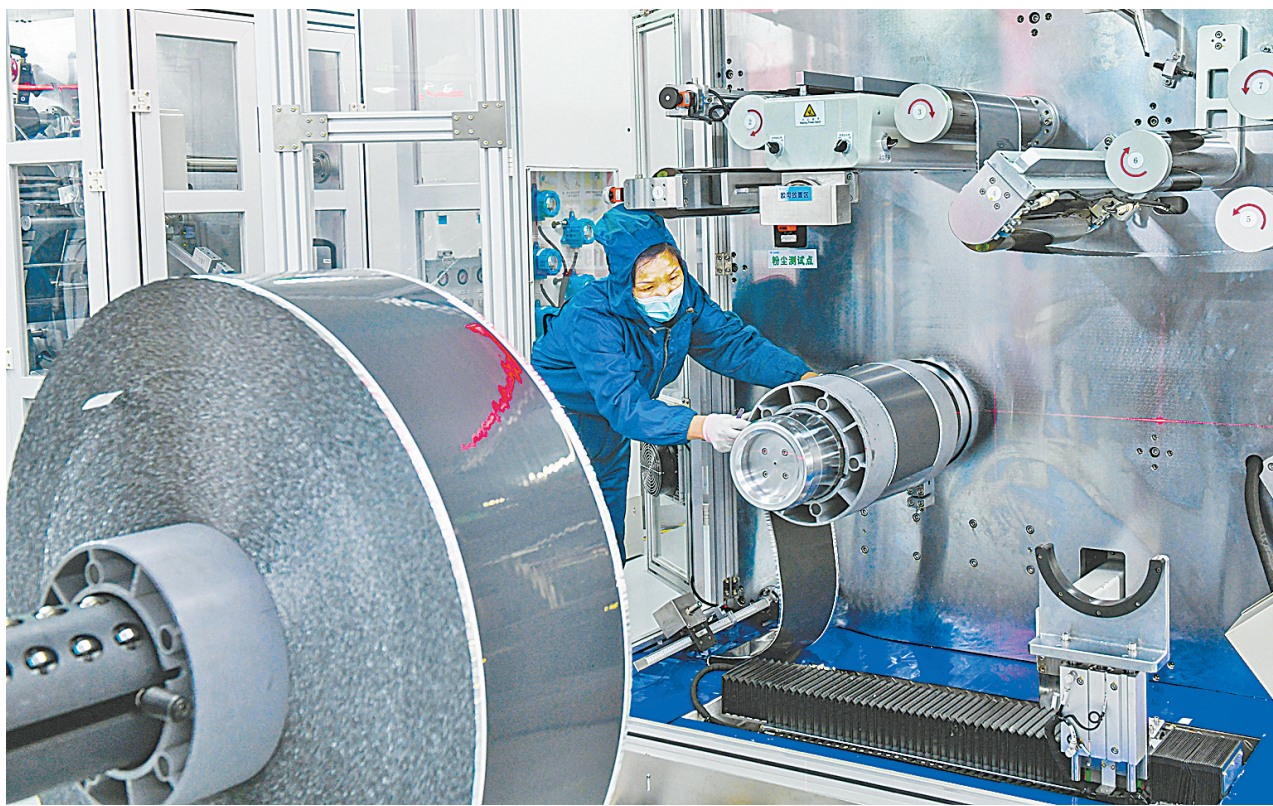
3月11日,多氟多年产8G瓦时锂离子电池项目生产线工人在安放锂电池生产材料。该项目是我市“三十工程”十大工业项目之一,总投资20.5亿元,目前项目一期已经建成投产,待项目全部竣工后预计可实现年销售收入80亿元、利税1.6亿元,增加就业岗位1200个,形成产业集聚效应,加速我市工业转型升级。 本报记者 刘金元 摄
