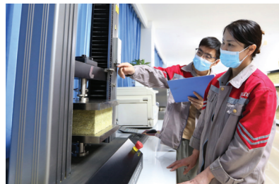
工作人员在做抗拉、抗压试验。
