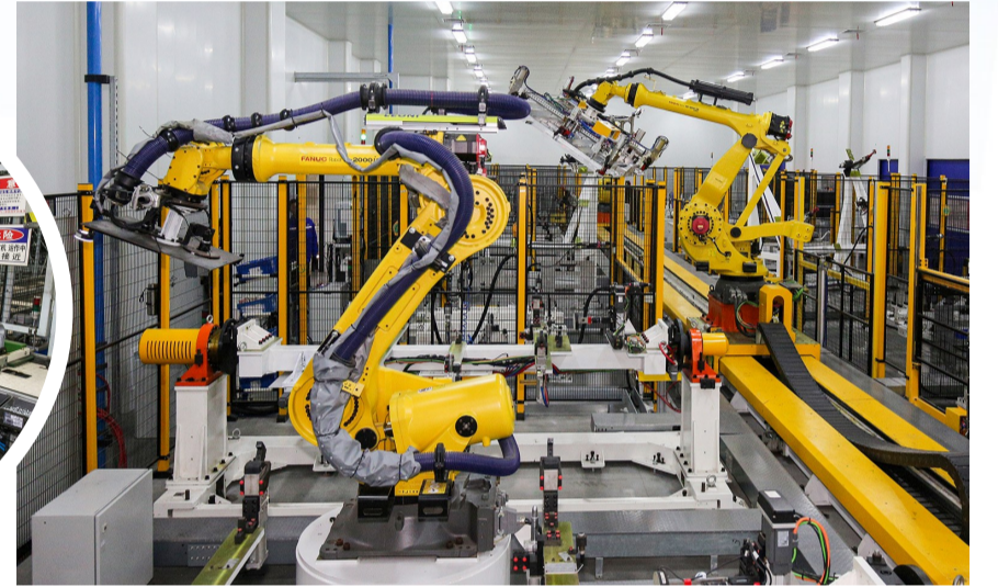
凌云电池PACK项目智能化车间
