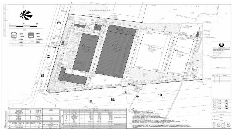
总平面图
