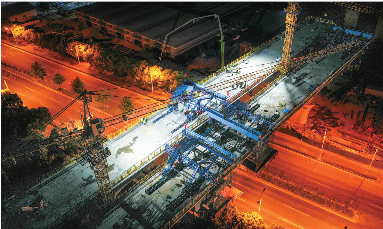
7月6日凌晨,位于松江区的沪苏湖铁路青浦特大桥斜塘桥段跨辰塔路连续梁完成合龙。图为施工现场。记者 蔡斌 摄
