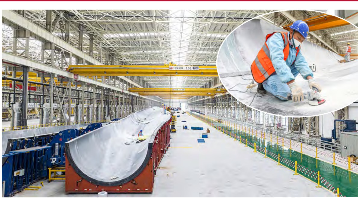
位于射阳港经济开发区的中车百米级超大叶片智造基地总投资达35亿元,规划建筑面积超13万平方米。当前,该项目112米、123米叶片生产线已进场生产。图为该项目生产车间内忙碌的生产场景。
